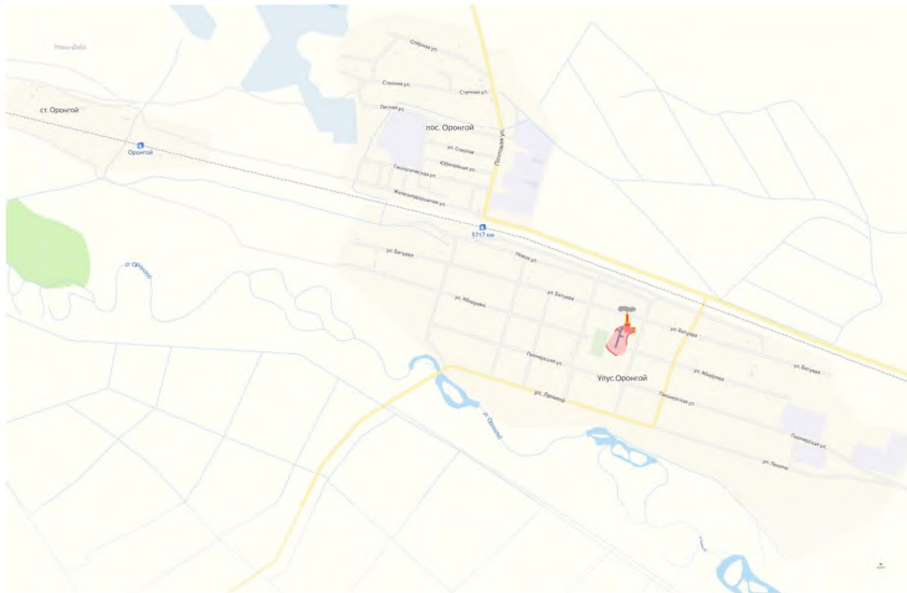
Рисунок 3. Зона действия источника теплоснабжения с. Оронгой.
