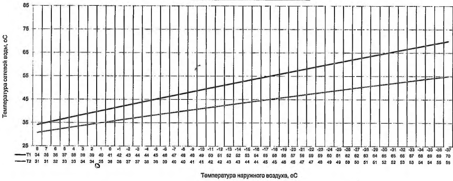
Рисунок 2. Температурный график отпуска тепловой энергии в сеть.
