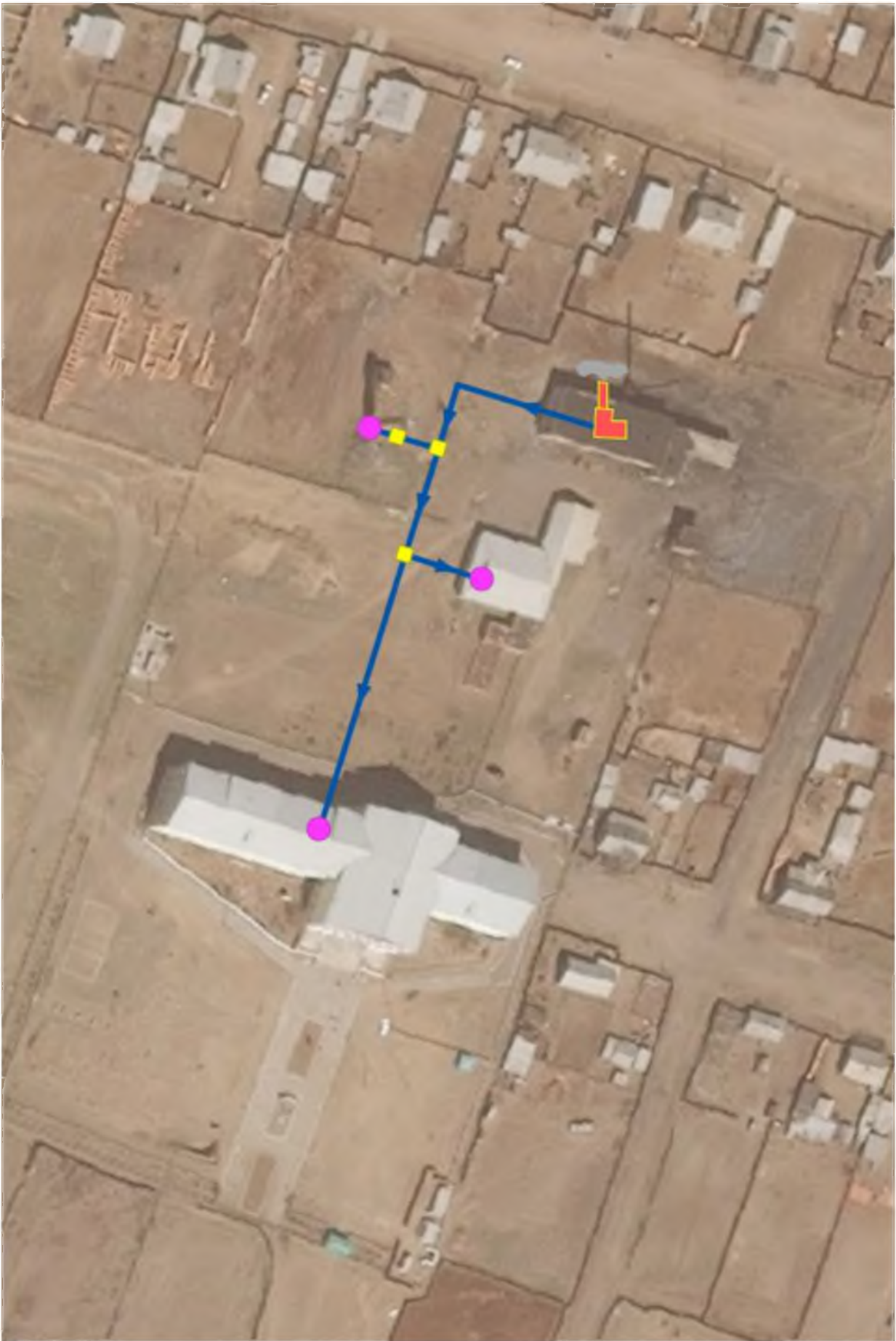
Рисунок 1. Графическая схема тепловых сетей котельной с. Оронгой.
